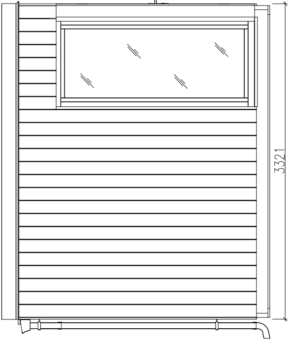
Left 1:50
